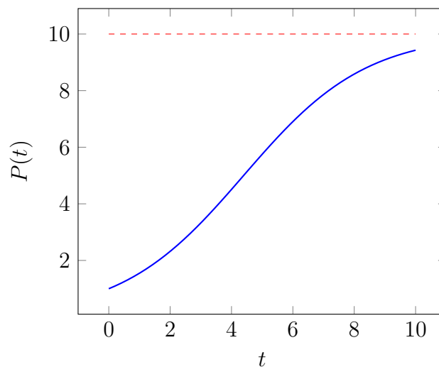
شکل ۹-۱: منحنی لجستیک (ظرفیت محدود)
