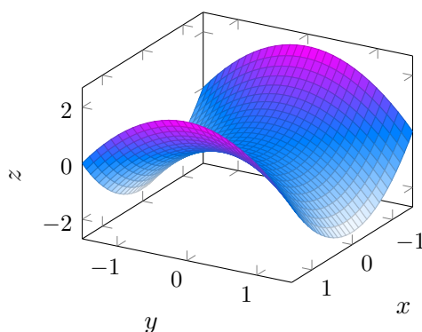
شکل ۱-۲: نقطه زینی f(x, y) = x^2 - y^2
