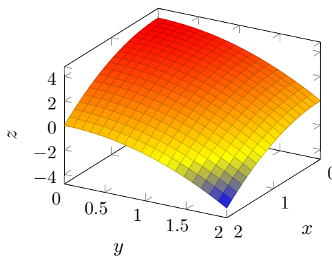
شکل ۸-۱: حجم زیر سهمی وار
