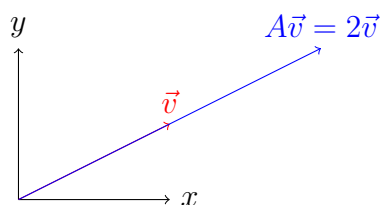
شکل ۶-۱: اثر ماتریس بر بردار ویژه (کشش)
