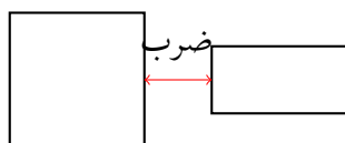
شکل ۴-۱: ضرب ماتریس A_{2 \times 2} در B_{2 \times 1}
