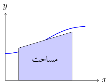
شکل ۷-۱: انتگرال معین به عنوان مساحت
