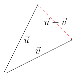
شکل ۳-۱: جمع و تفریق بردارها در صفحه
