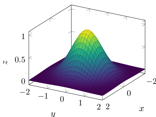
شکل ۱-۱: سطح تابع f(x, y) = e^{-(x^2+y^2)} (قله مرکزی)
